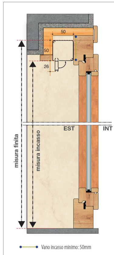
Sezione verticale
