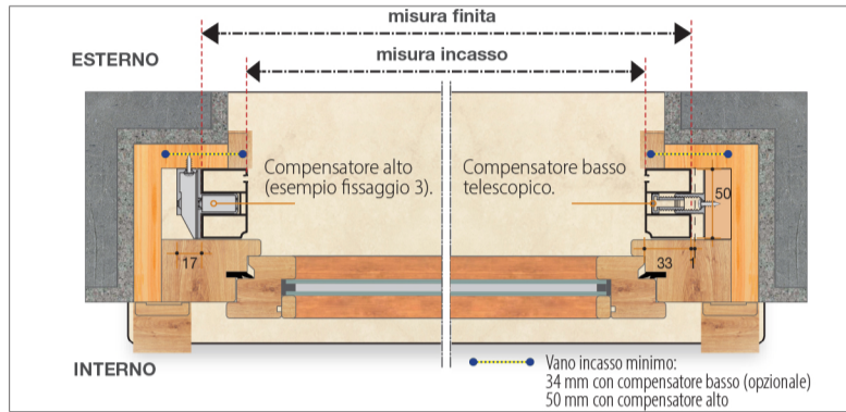
Sezione orizzontale
